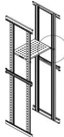
Sabit rafların arka montaj görünüşü
