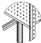
Sabit rafların ön montaj görünüşü
