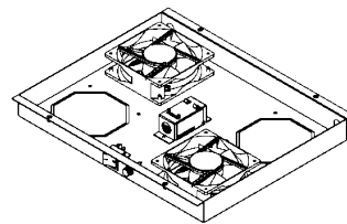
Perspektif Görünüş
