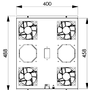
Üst Görünüş
