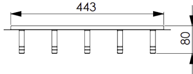
Üst Görünüş
