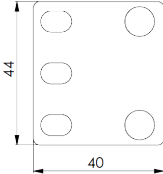
Ön Görünüş
