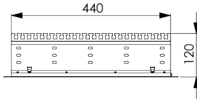
Üst Görünüş
